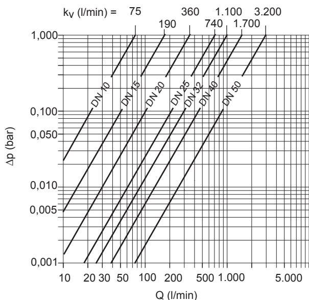
Диаграмма падения давления (ориентировочные значения для H 2 O, 20 °C)
